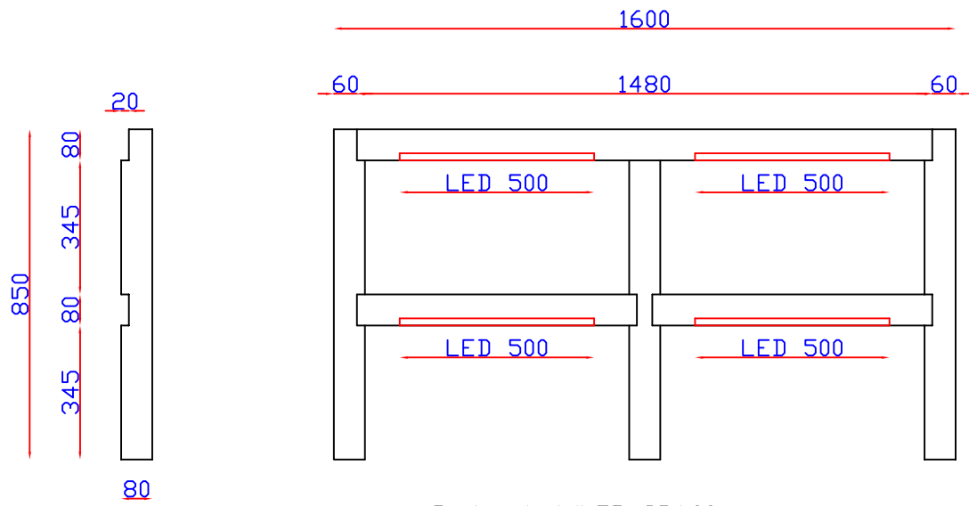
Badmeubel/LED SPA60
